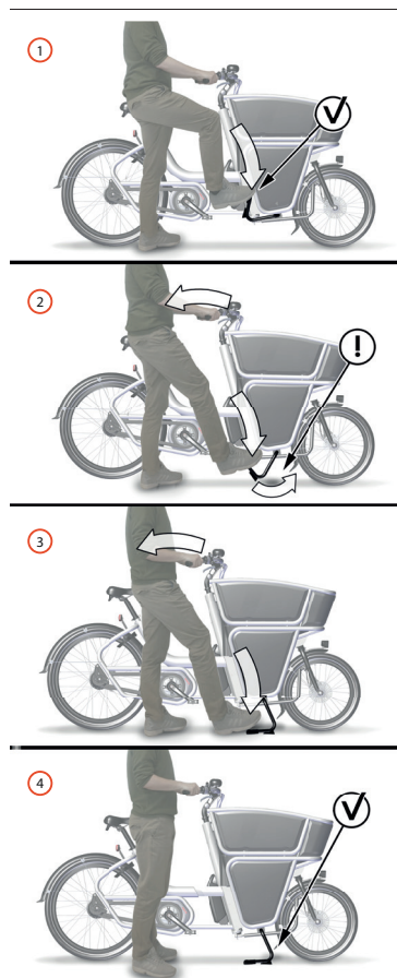
Abbildung 23 : Einklappen des Fahrradständers
