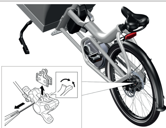
Image 38 : Retrait des plaquettes de frein afin de vérifier leur état d'usure
