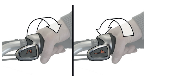
Afbeelding 25: Schakelen naar een lichtere (lagere) of zwaardere (hogere) versnelling
