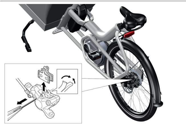
Afbeelding 38: Verwijderen van de remblokjes om ze op slijtage te controleren
