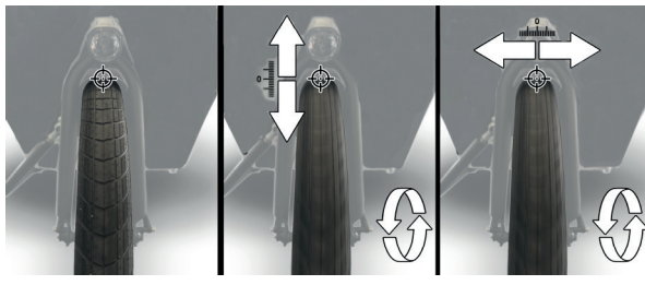
Abbildung 34 : Prüfen des Seitenschlags
