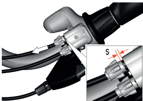
Afbeelding 39: Kabelspeling controleren
