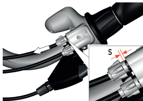
Image 39 : Vérification du jeu du câble
