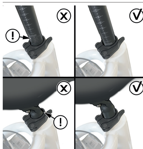
Image 7 : Insertion maxi et mini de la tige de selle
