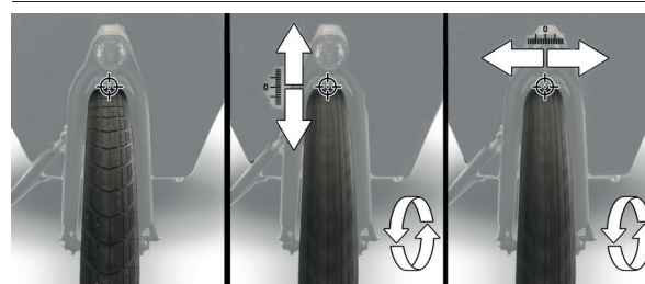
Image 34 : Vérification du décalage de la roue
